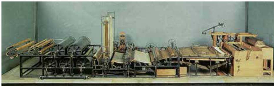
6. Modello di una delle prime macchine per la fabbricazione di un foglio continuo di carta, avvolto su bobine.
