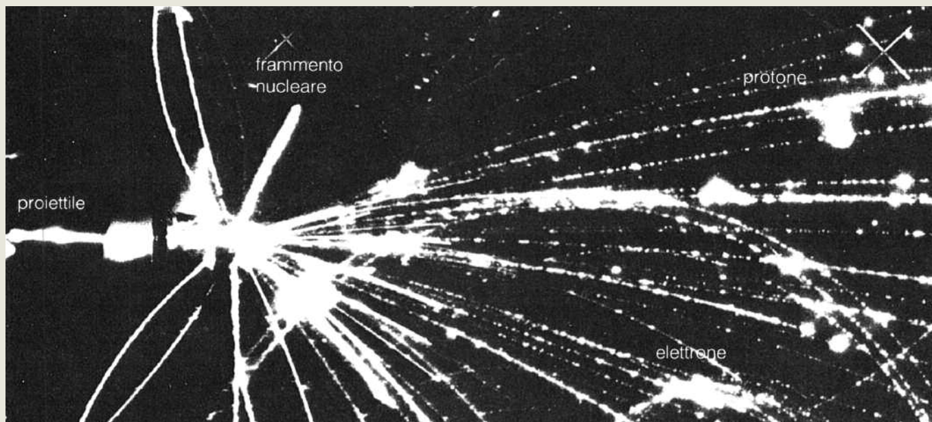
Fig. a. Dalla collisione di un nucleo di argo 40, la cui energia cinetica era di 72 miliardi di elettronvolt, con un nucleo di atomo di piombo, si vedono, nella foto e nello schema, le tracce di protoni e di due elettroni. (@ Lawrence Berkeley Laboratory, California).
