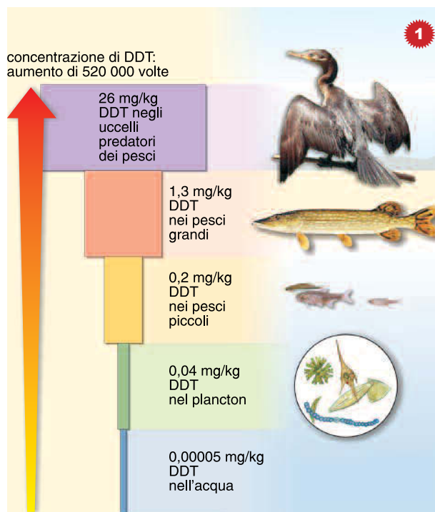
Fig. 1. Lo schema rappresenta il processo di bioaccumulo del DDT nella catena alimentare. Il DDT presente in minime quantità nell'acqua, attraverso la catena alimentare arriva a concentrarsi ben 520 000 volte nei tessuti del cormorano.
