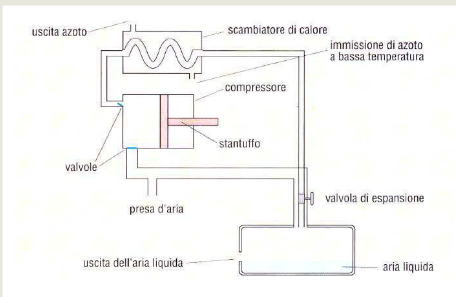
1. Schema del processo Linde per la liquefazione dell'aria.
