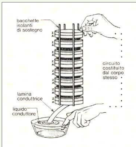
1. (a) e (b) Schemi delle prime pile di Volta.
