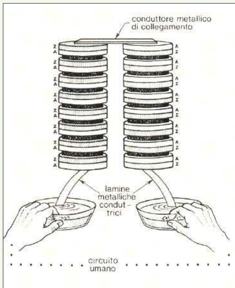
1. (a) e (b) Schemi delle prime pile di Volta.
