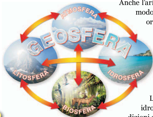
Fig. 1. Una rappresentazione del sistema Terra.
