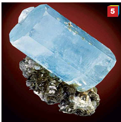
Fig. 5. Cristallo di acquamarina su muscovite.
