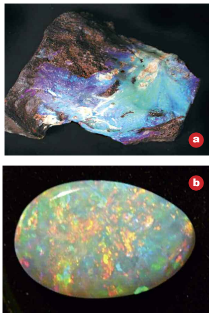
Fig. 7. a. Opale grezzo. b. Opale lavorato e lucidato con la caratteristica iridescenza.
