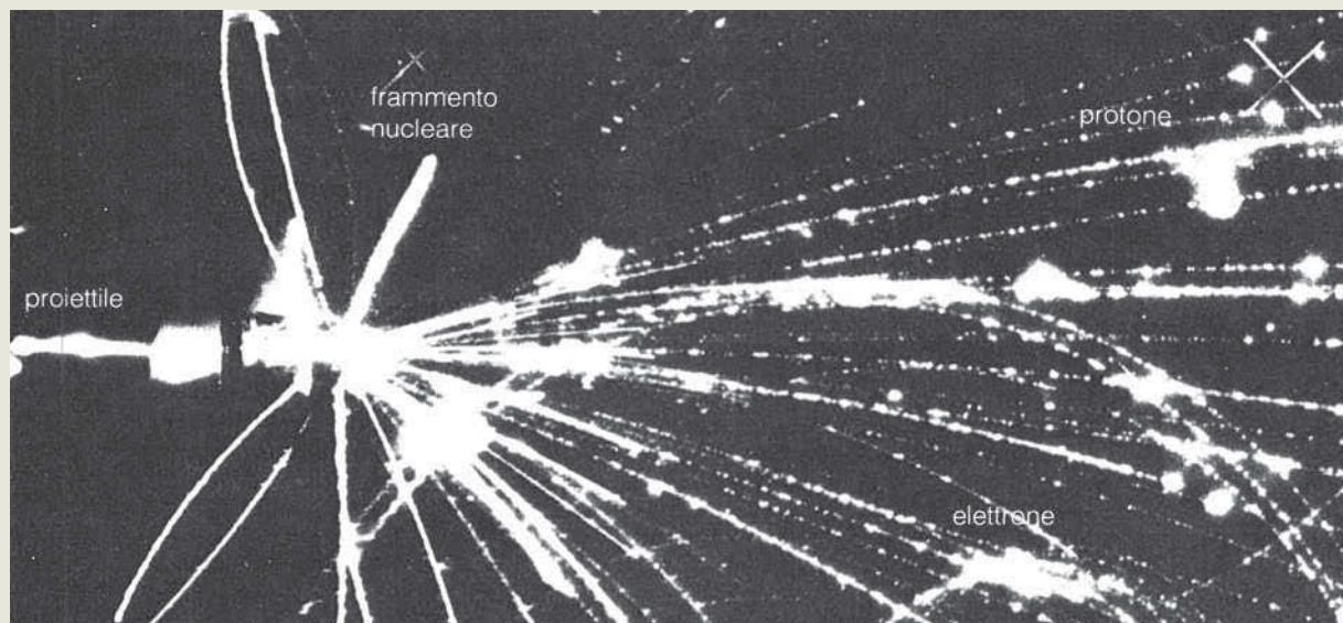
1. Dalla collisione di un nucleo di argo 40, la cui energia cinetica era di 72 miliardi di elettronvolt, con un nucleo di atomo di piombo, si vedono, nella foto e nello schema, le tracce di protoni e di due elettroni.
