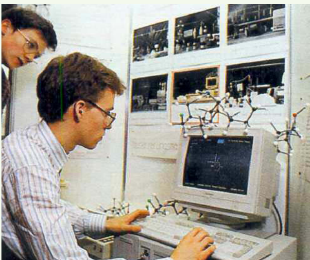
3. Applicazione dell'informatica alla chimica.
