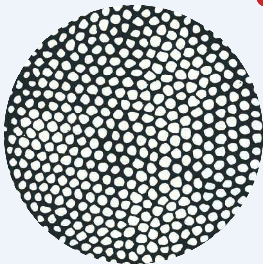
1. INSTABILITÀ DI BÉNARD. La figura rappresenta una vista dall'alto di uno strato liquido piuttosto sottile riscaldato dal basso. Quando il gradiente termico è piccolo il calore viene trasportato per conduzione e il liquido mostra una perfetta omogeneità statica. Quando però il gradiente termico supera un certo valore si produce un trasporto di calore per convezione che produce un ordinato arrangiamento di cellette di convezione corrispondenti ad uno stato di equilibrio dinamico.
