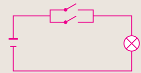
Circuito OR
