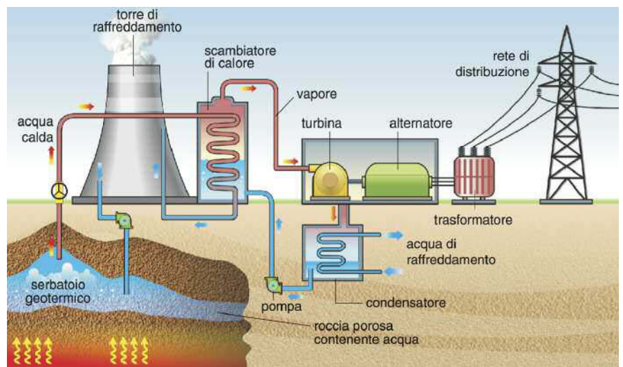
Fig. 1. Schema di un campo geotermico e di un impianto tipo per il suo sfruttamento: il serbatoio geotermico è costituito da uno strato di roccia porosa, contenente acqua a circolazione sotterranea, compreso tra due strati di roccia impermeabile, di cui quello inferiore a contatto con il magma di una sottostante camera magmatica.
