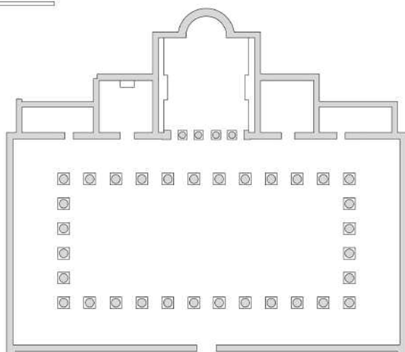
Sabratha, Libia, pianta della basilica, II metà del I sec. d.C.
