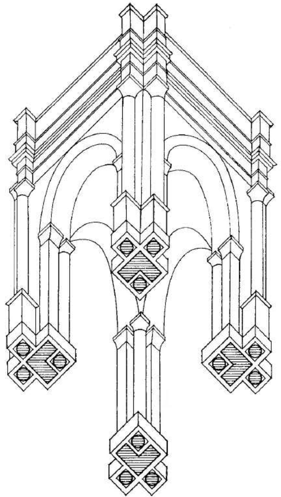
Leptis Magna, Arco di Traiano, 109-110. Assonometria.
